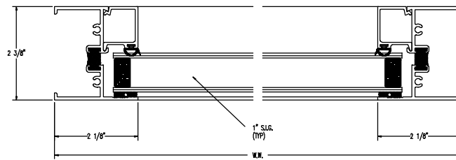
4 FIXED JAMB
