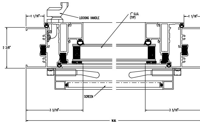
6 LOCK JAMB
